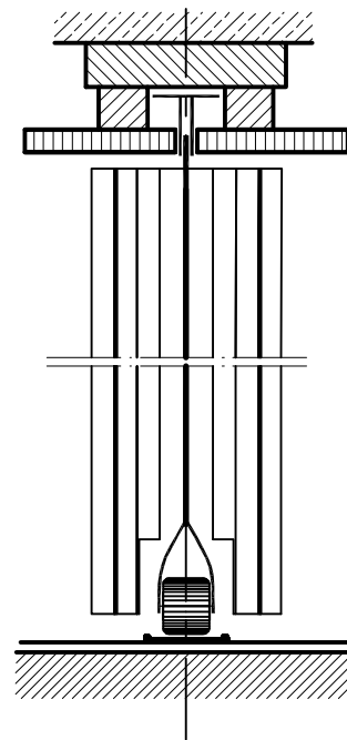
BOTTOM ROLLER
